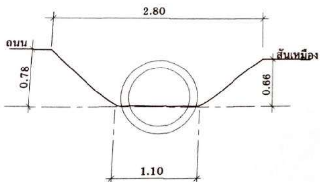
รูปตัดตามขวางลำเหมือง Sta. 0+000
