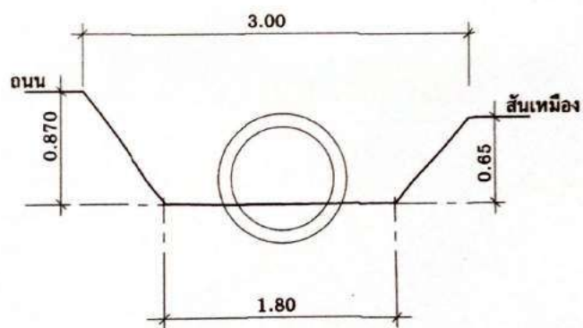
รูปตัดตามขวางลำเหมือง Sta. 0+025
