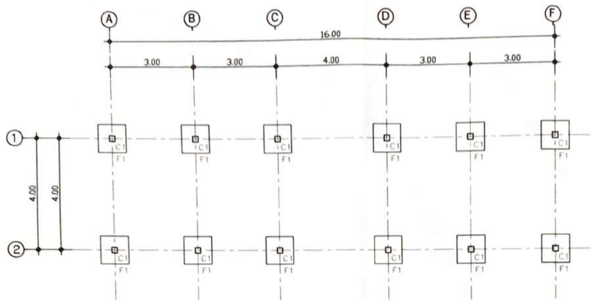
แปลนฐานราก เสา มาตราส่วน 1:100
