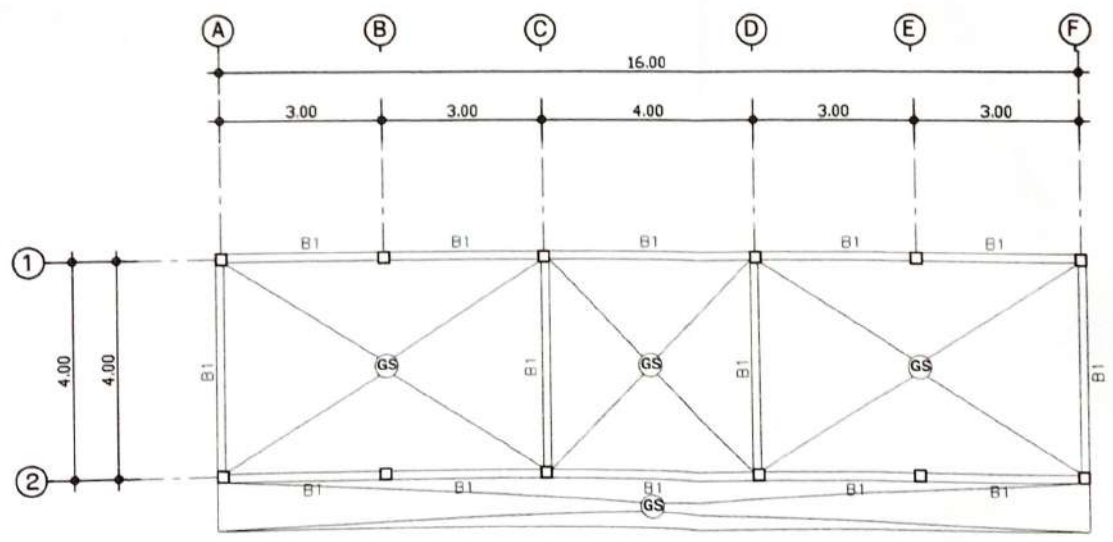
แปลนคานาพื้น มาตราส่วน 1:100
