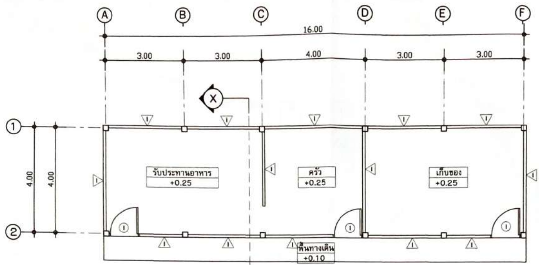
แปลนพื้น มาตราส่วน 1:100
