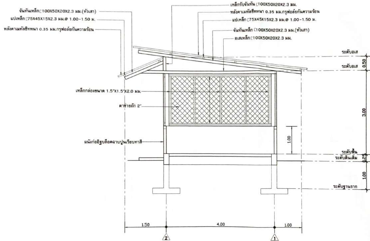
รูปตัดแนวขวาง มาตราส่วน 1:50
