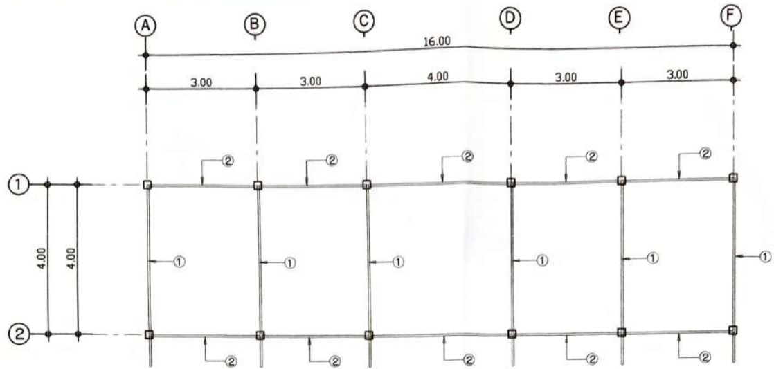
โครงสร้างหลังคา มาตราส่วน 1:100
