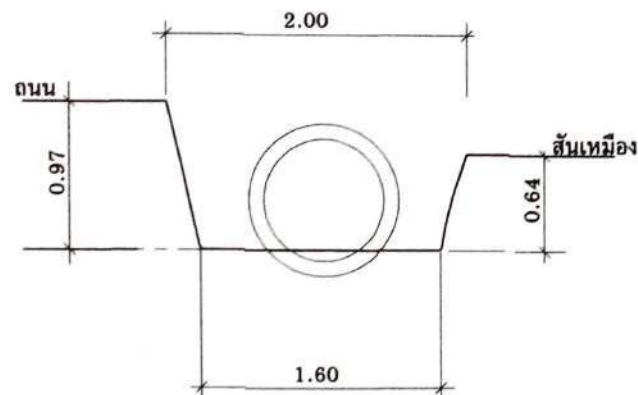
รูปตัดตามขวางลำเหมือง Sta. 0+100
