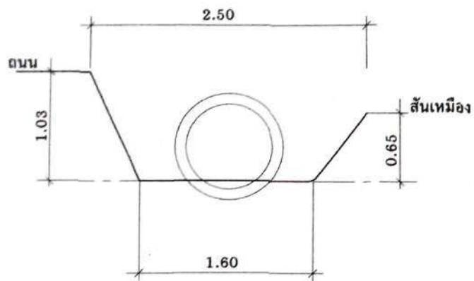
รูปตัดตามขวางลำเหมือง Sta. 0+075
