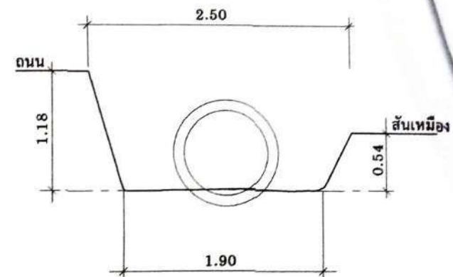
รูปตัดตามขวางลำเหมือง Sta. 0+125
