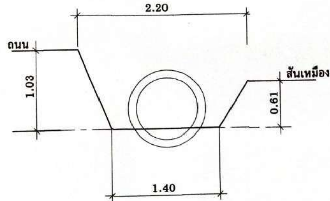
รูปตัดตามขวางลำเหมือง Sta. 0+025
