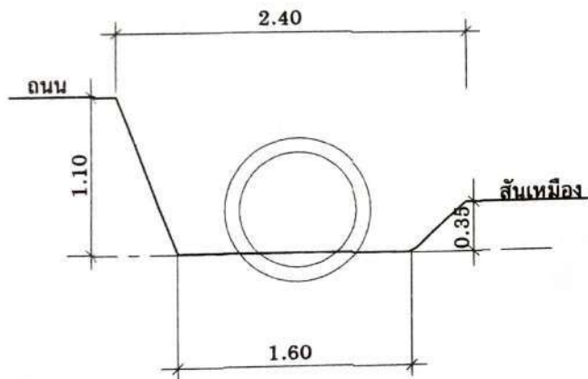
รูปตัดตามขวางลำเหมือง Sta. 0+000
