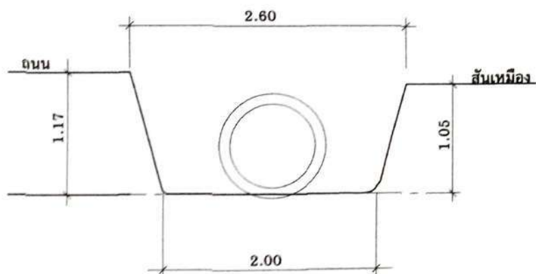
รูปตัดตามขวางลำเหมือง Sta. 0+150
