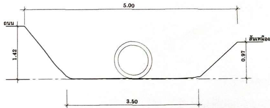
รูปตัดตามขวางลำเหมือง Sta. 0+180
