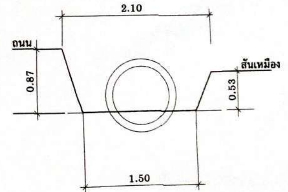
รูปตัดตามขวางลำเหมือง Sta. 0+050
