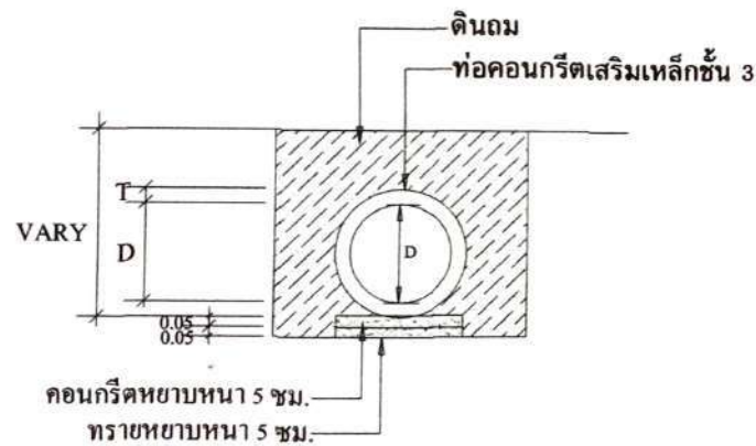
รูปตัดทางขวางที่ 3
