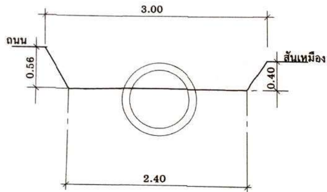
รูปตัดตามขวางลำเหมือง Sta. 0+075
