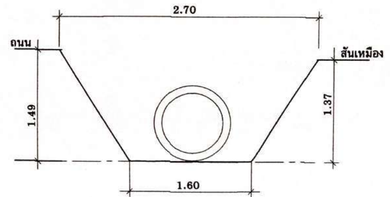
รูปตัดตามขวางลำเหมือง Sta. 0+177
