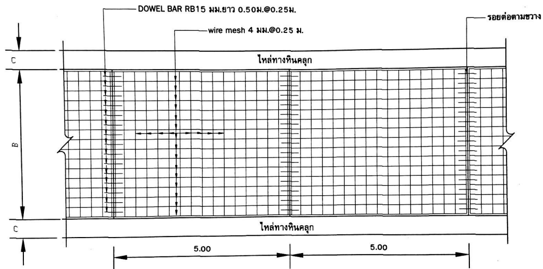
รูปแปลนผิวดำรงคอนกรีตเสริมเหล็ก
