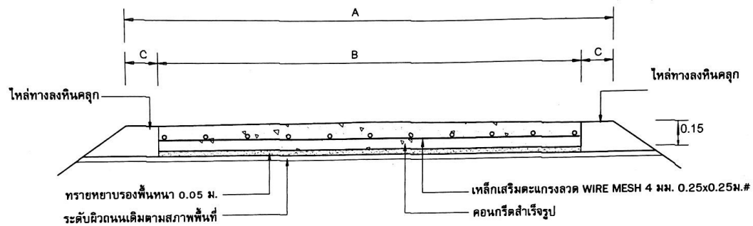
รูปตัดตามขวาง A
