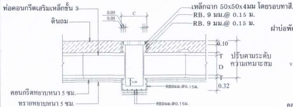
รูปตัดทางยาวที่ 1
