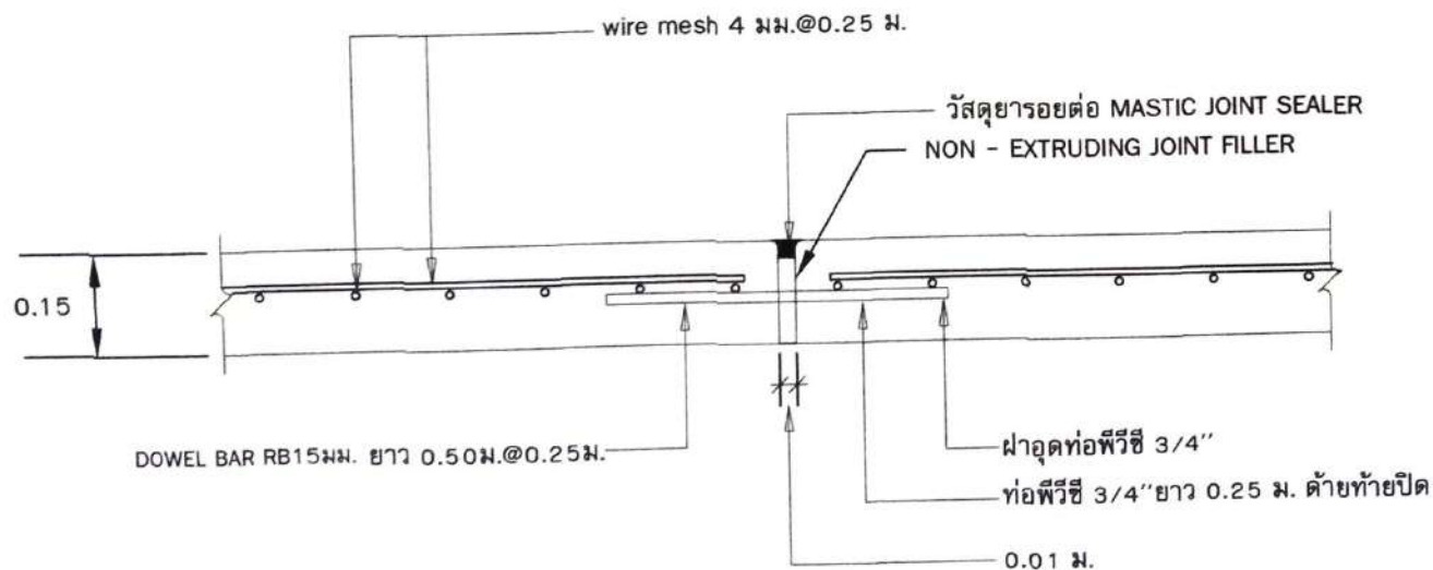
ขยายรอยต่อ EXPANSION JOINT ทุกระยะ 50 เมตร
