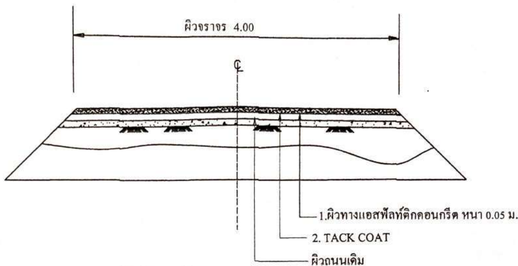
รูปตัดโครงสร้างถนน
