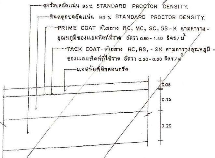
รายละเอียด ASPHALTIC CONCRETE not to scale
