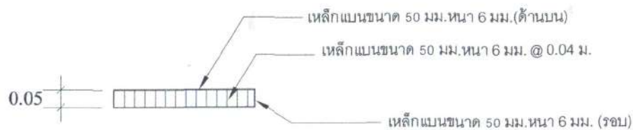
ขยายรูปตัดฝาบ่ปิดบ่อพัก
