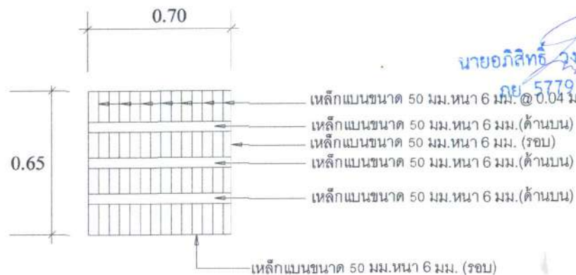
ขยายรูปฝาบ่ปิดบ่อพัก
